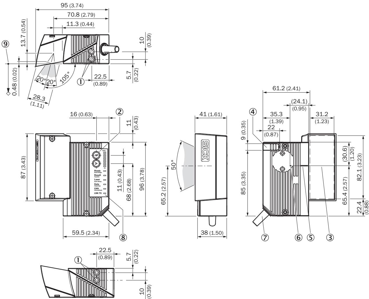
Rysunek wymiarowy CLV63x/64x/65x Standard, wahliwe lustro
