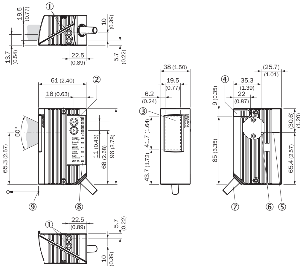
Rysunek wymiarowy CLV63x/64x/65x Standard, od strony czoła
