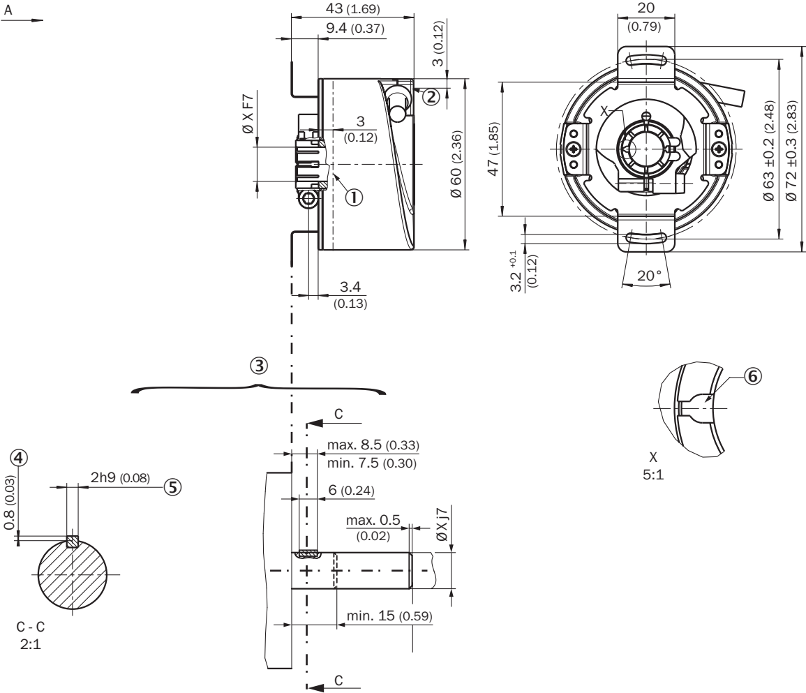
Rysunek wymiarowy Otwór przelotowy, przewód
