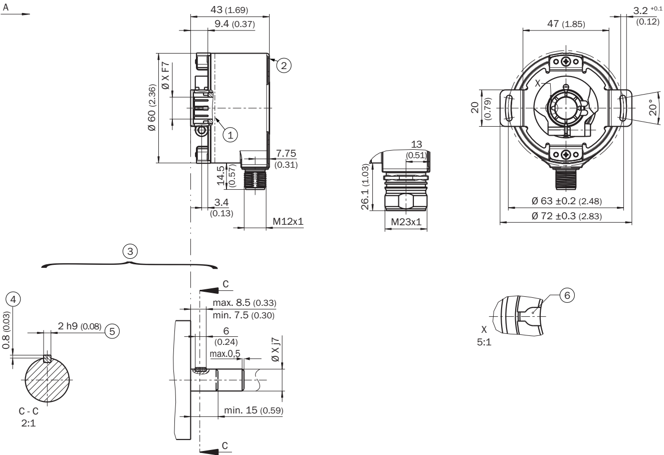
Rysunek wymiarowy Otwór przełotowy, wtyk promieniowy M12 i M23
