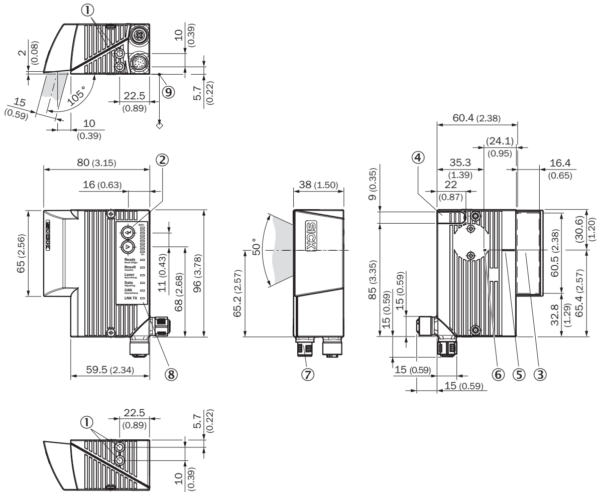
Rysunek wymiarowy CLV63x/64x Ethernet, z boku
