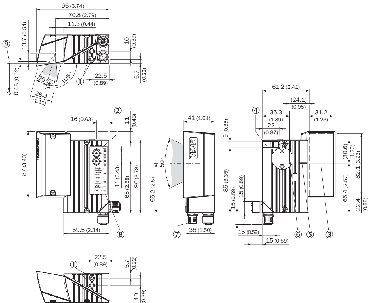
Rysunek wymiarowy CLV63x/64x/65x, JEF3xx, JEF5xx, Ethernet, wahliwe lustro
