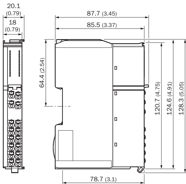
Rysunek wymiarowy EMSS1, HAND1, OSSD1, OSSD2, TIME1
