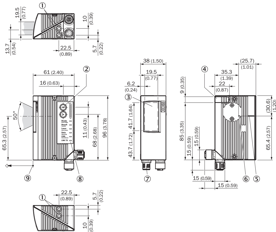
Rysunek wymiarowy CLV63x/64x/65x, JEF3xx, JEF5xx, Ethernet, od strony czoła
