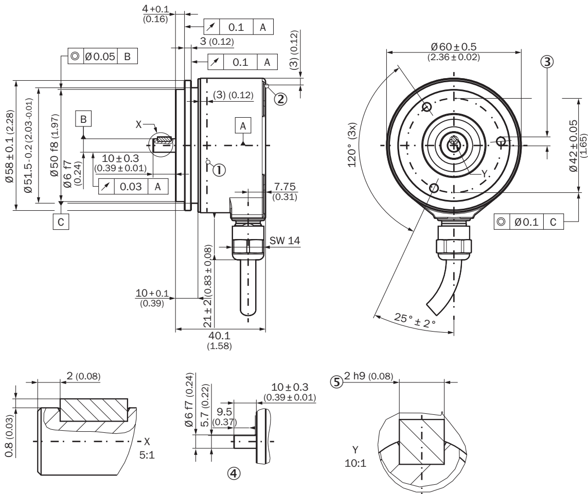
Rysunek wymiarowy Wałek, mocowanie na serwokolnierzu, przewód promieniowy
