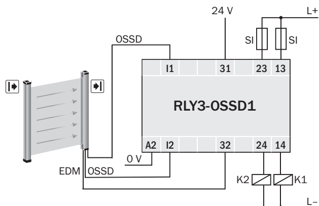
RLY3-OSSD1 do optoelektronicznej kurtyny bezpieczeństwa z monitorowaniem urządzeń zewnętrznych
