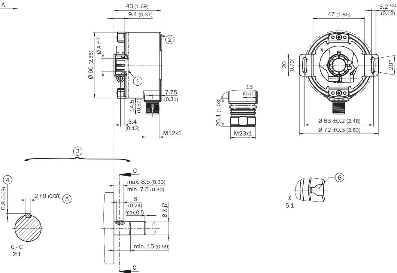
Rysunek wymiarowy Otwór przelotowy, wtyk promieniowy M12 i M23
