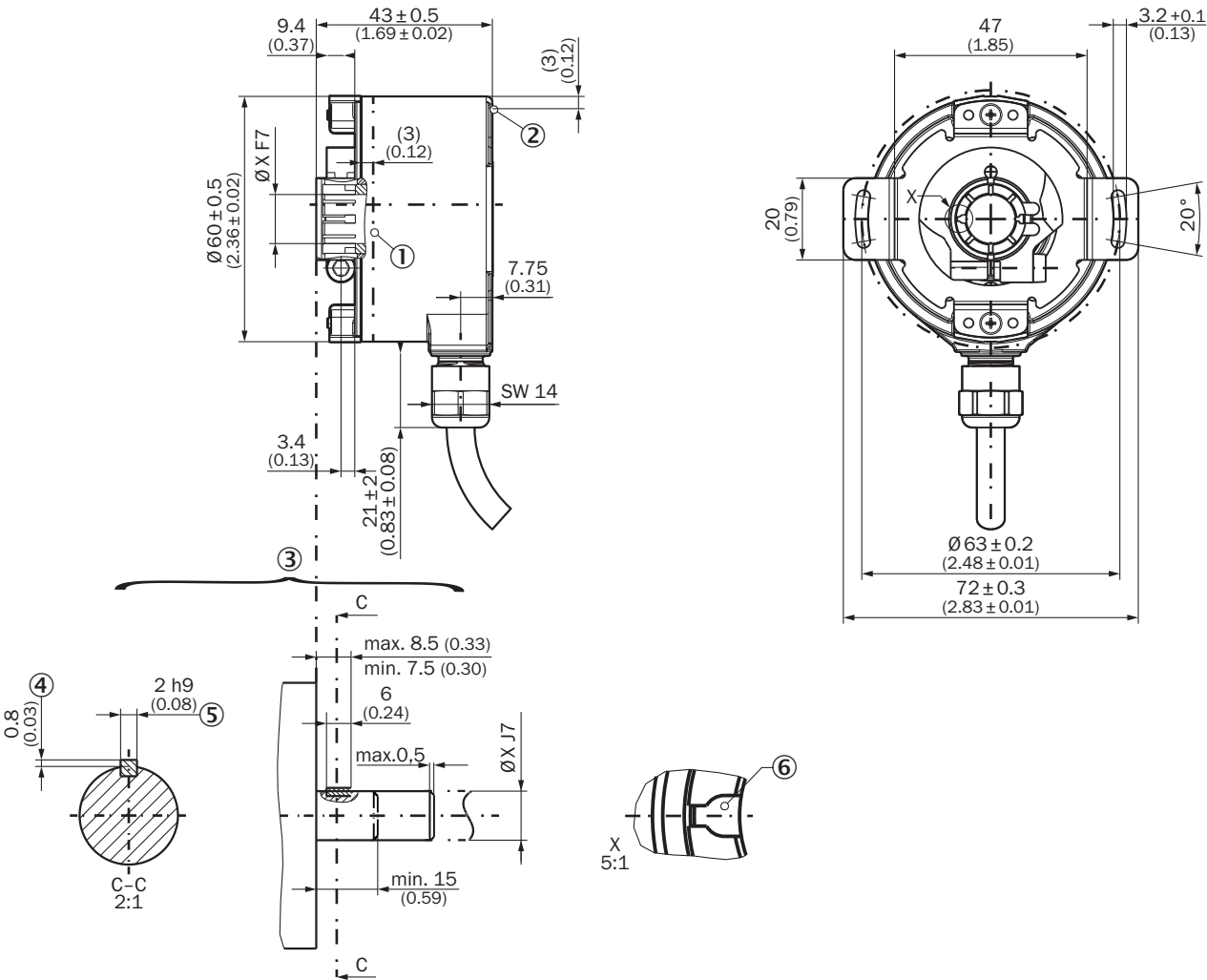
Rysunek wymiarowy Otwór przełotowy, przewód promieniowy
