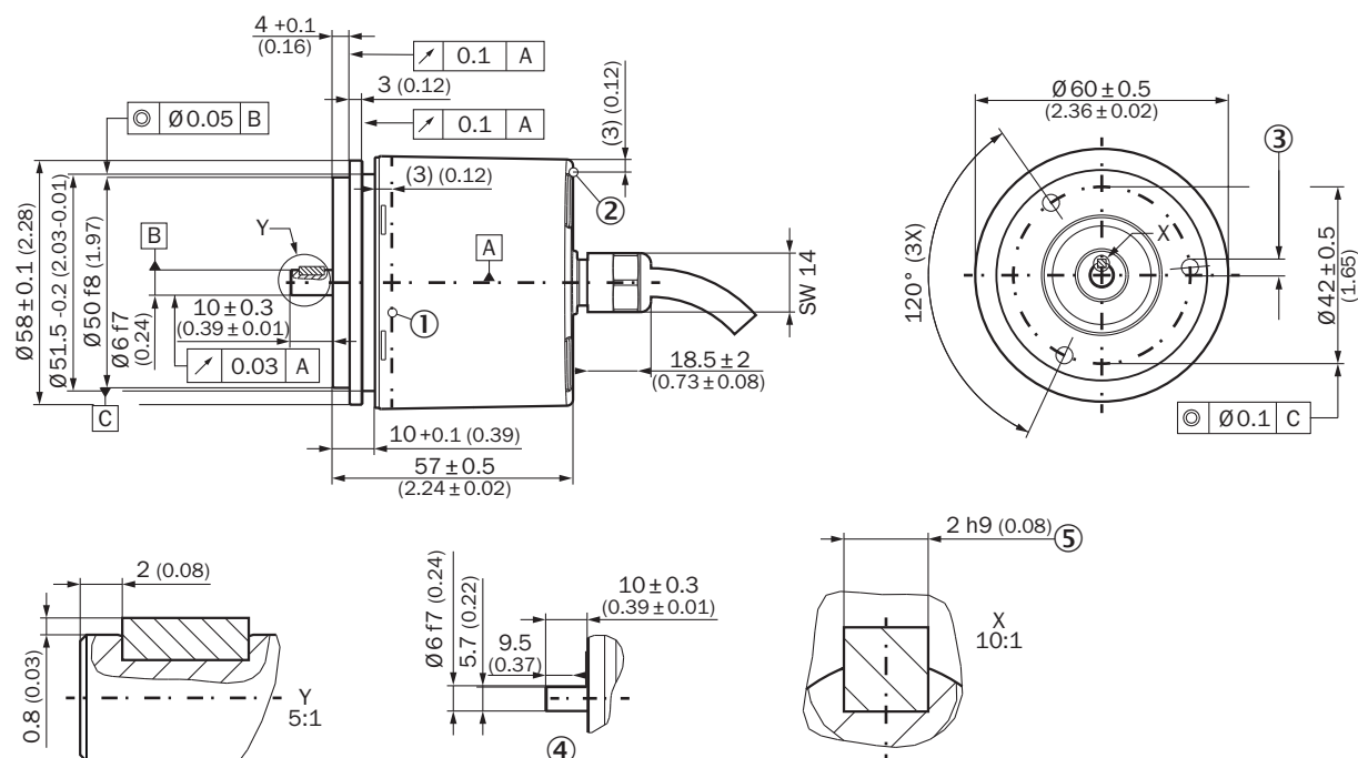
Rysunek wymiarowy Wałek, mocowanie na serwokołnierzu, przewód osiowy
