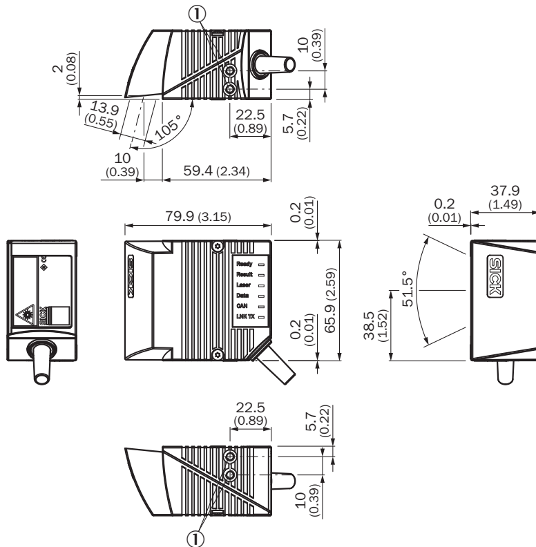
Rysunek wymiarowy CLV62x Standard, z boku
