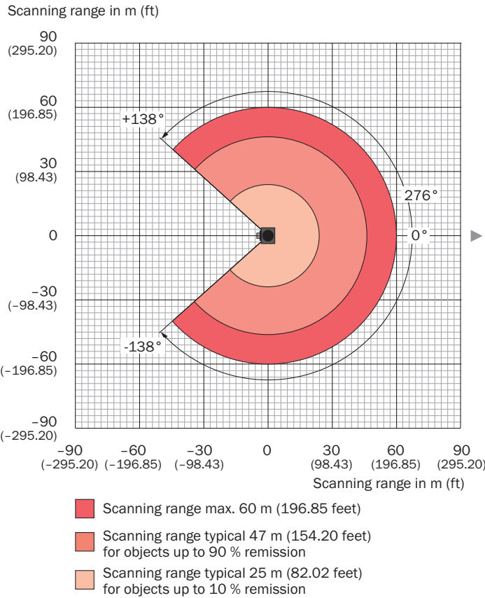
Wykres obszaru roboczego Zakres roboczy picoScan150 Prime-1
