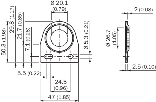
Rysunek wymiarowy
