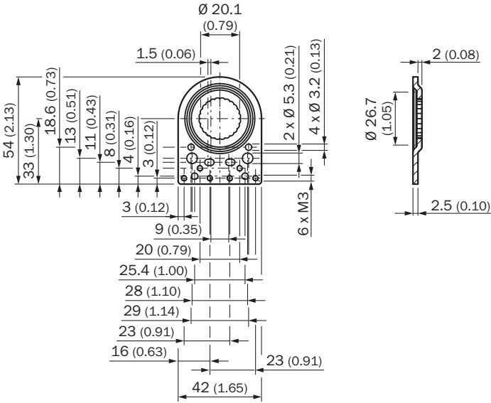
Rysunek wymiarowy
