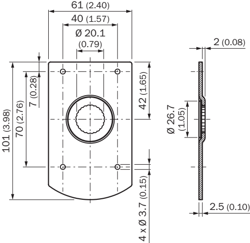
Rysunek wymiarowy
