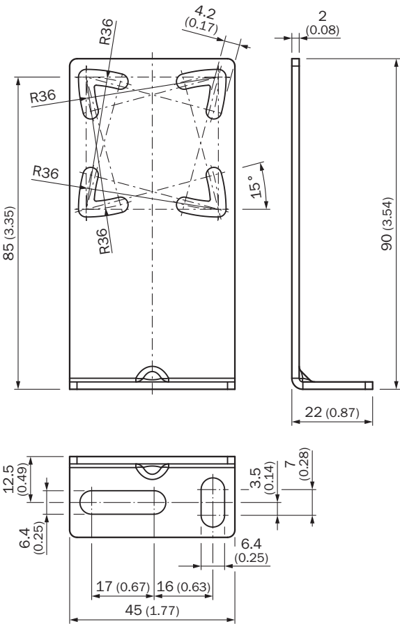
Rysunek wymiarowy
