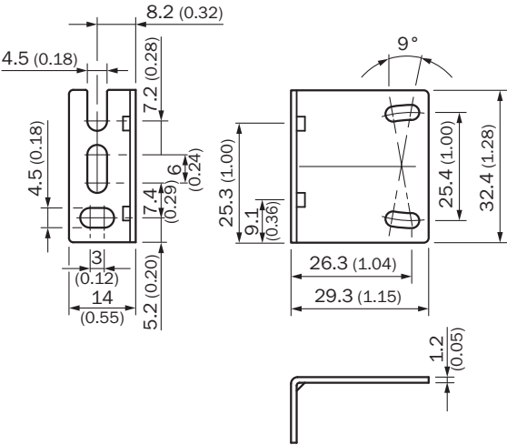
Rysunek wymiarowy
