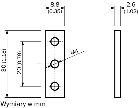
Rysunek wymiarowy
