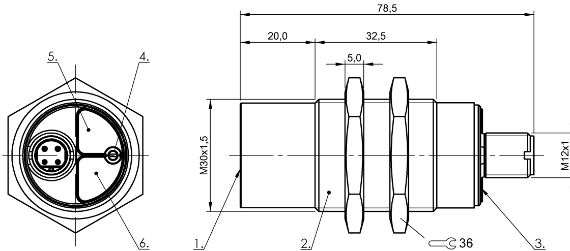
1) powierzchnia aktywna 2) Obudowa 3) Pokrywa 4) Potencjometr 5) Napięcie robocze LED 6) Wskazanie funkcji LED
