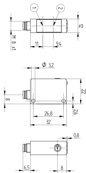
Maßangaben in mm / All dimensions in mm / Mesures en mm ① = Sendediode / Transmitter diode / Diode émettrice ② = Empfangsdiode / Receiver diode / Diode réceptrice Schraube / Screw / Vis M3 = 0,5 Nm
