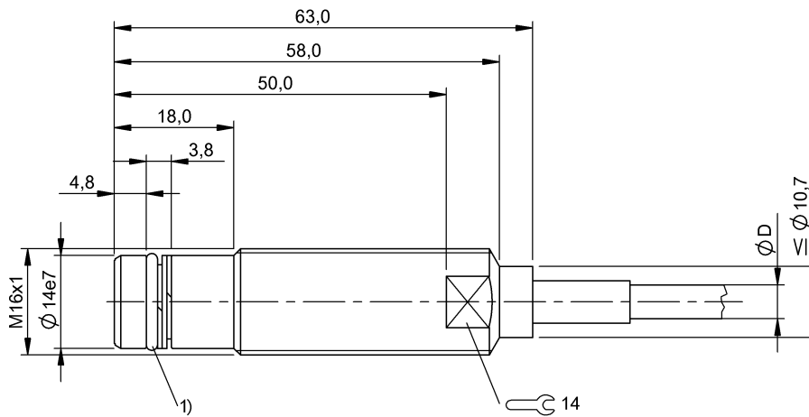
1) O-ring z pierścieniem oporowym
