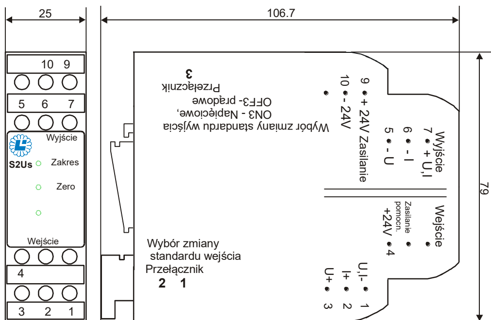
Szkic obudowy
