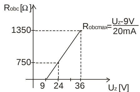
Rys.1. Sposób Wyznaczenia rezystancji obciążenia separatora S3
