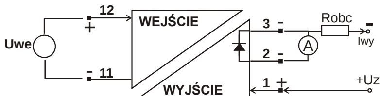
Rys. 2e. Podłączenie sygnału napięciowego z pomiarem prądu wyjściowego.
