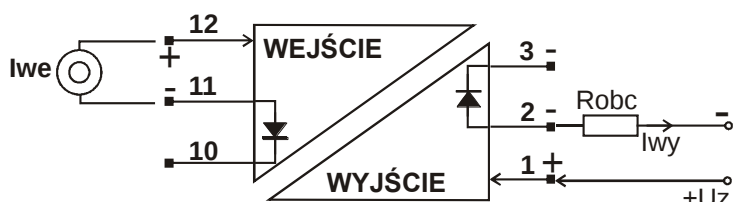
Rys. 2b. Podłączenie sygnału prądowego bez pomiaru prądu.
