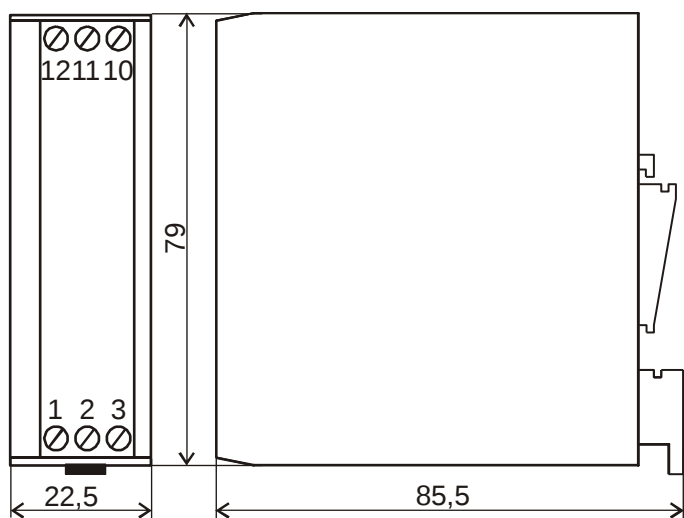
Rys. 2a. Rozkład zacisków podłączeniowych separatora S3.
