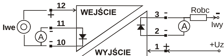
Rys. 2c. Podłączenie sygnału prądowego z pomiarem prądu wejściowego i wyjściowego.
