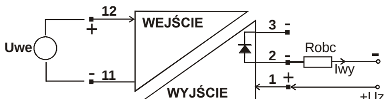
Rys. 2d. Podłączenie sygnału napięciowego bez pomiaru prądu wyjściowego.
