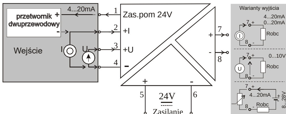
Rys.1 Schemat funkcjonalny ilustrujący możliwe opcje wykonañ.
