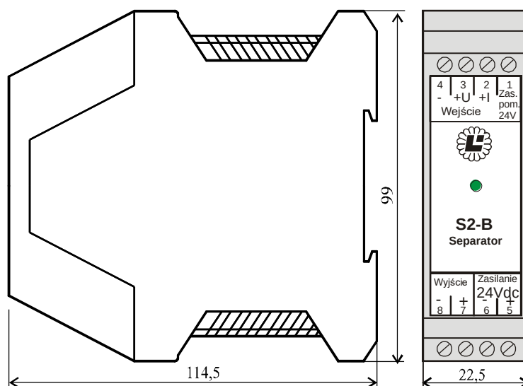
Rys.2 Rysunek mechaniczny obudowy z rozmieszczeniem zacisków.
