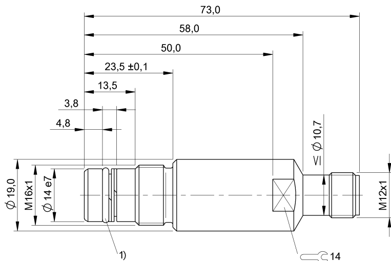
1) O-ring z pierścieniem oporowym
