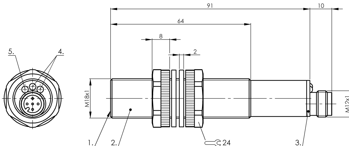
1) powierzchnia aktywna 2) Obudowa 3) Pokrywa 4) Wskazanie funkcji żółty 5) Wskaźnik Echo, zielony
