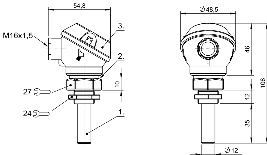
1) powierzchnia aktywna 2) Obudowa 3) Pokrywka
