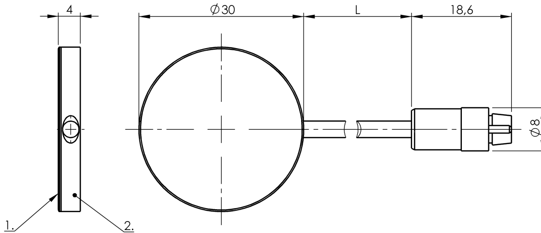
1) powierzchnia aktywna 2) Obudowa
