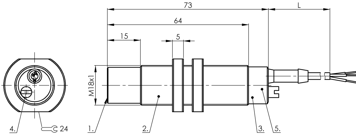
1) powierzchnia aktywna 2) Obudowa 3) Pokrywka 4) Potencjometr 5) Wskazanie funkcji LED
