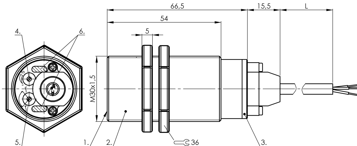
1) powierzchnia aktywna 2) Obudowa 3) Pokrywka 4) Potencjometr 5) Możliwość wyboru NO lub NC 6) Wskazanie funkcji LED
