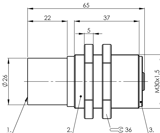
1) powierzchnia aktywna 2) Obudowa 3) Pokrywka
