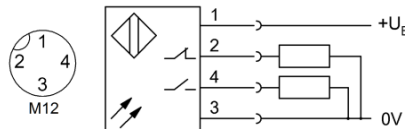
Bild 13: Steckerbild, Anschluss-Schaltbild
