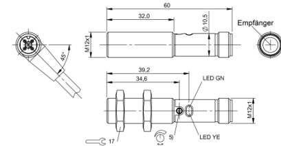
Bild 9: Abmessungen
