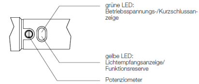
Bild 5: Anzeige- und Bedienelemente (bei BOS 12M-PA-RE10-..)
