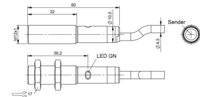
Bild 8: Abmessungen
