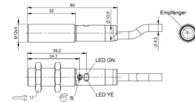
Bild 10: Abmessungen
