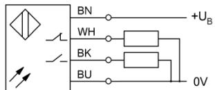
Bild 14: Anschluss-Schaltbild
