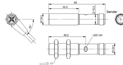
Bild 7: Abmessungen
