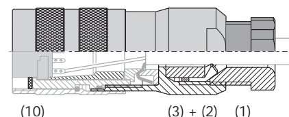
Bild 6: PG-Verschraubung montiert, Steckverbinder komplett
