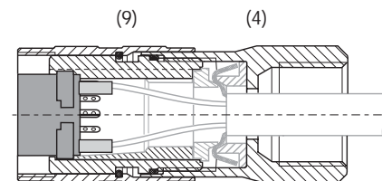
Bild 5: Vorderer Teil des Steckverbinders montiert
