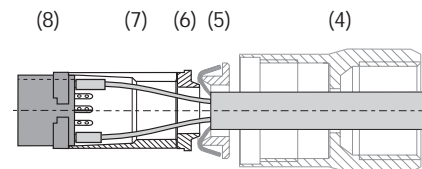
Bild 4: Adern angelötet, Distanzrohr (7) montiert
