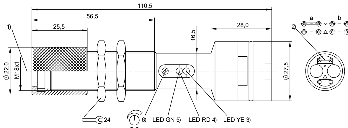
1) Oś optyczna 2) a= ciemny / b= jasny 3) Odbiór światła 4) Błąd 5) Stabilność 6) Sn
